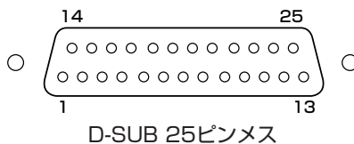
D-SUB 25ピンメス
