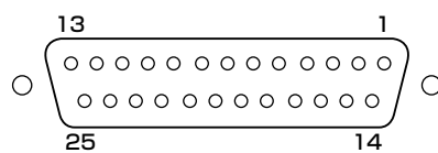
D-SUB 25ピンメス
