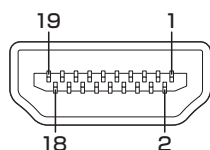
コネクタ図
