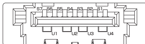
コネクタ図
