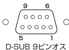
コネクタ図
