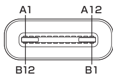
コネクタ図
