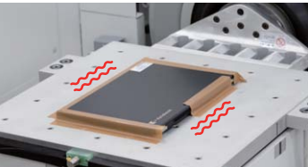
電車や車移動などで振動を受けることを想定し、テーブルをXYZの3方向それぞれで振動させてPCが壊れないか評価します。
