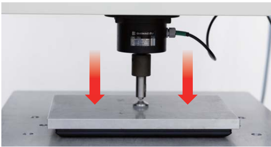
満員電車など、液晶カバーに圧がかかることを想定し、液晶カバー全面に100kgfの加圧を与え、液晶パネルが割れないことを確認しています。 * モデルによっては200kgf加圧。
