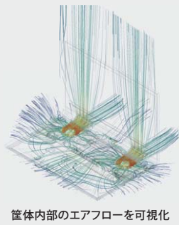
筐体内部のエアフローを可視化
