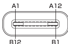
コネクタ図
