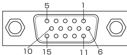
15ピン ミニD-sub 3段
