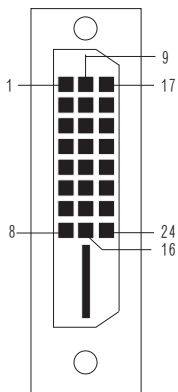
コネクタ図
