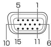
コネクタ図
