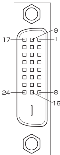
コネクタ図
