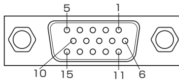
D-SUB15 ピンメス (3列タイプ)
